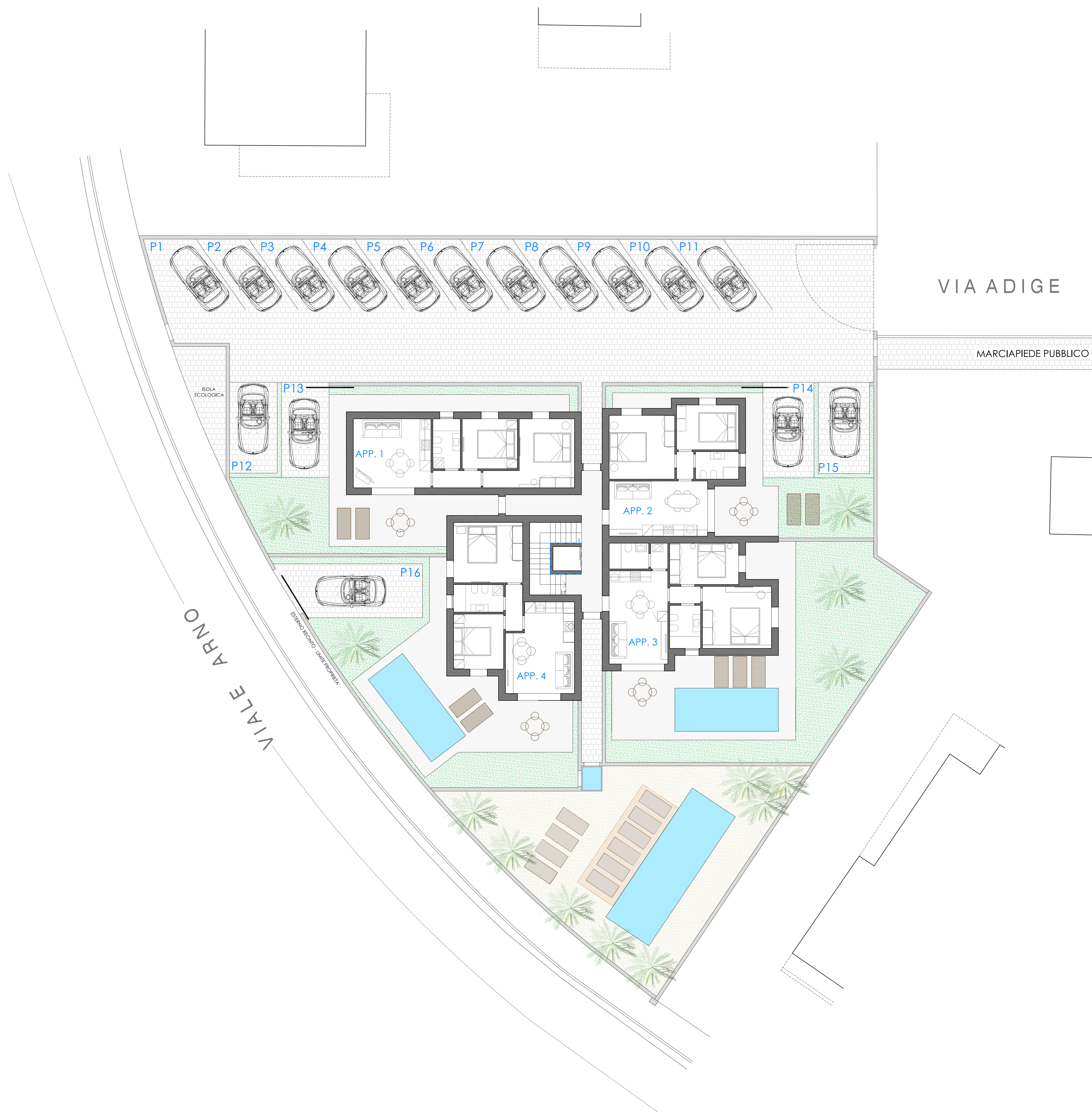
Piano TERRA_Scala 1:100
